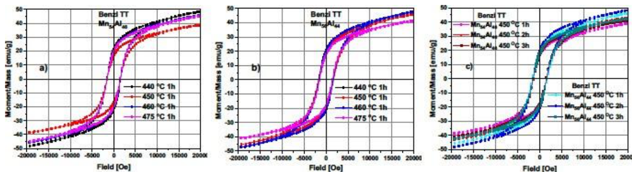
Fig. 12. Curbele de histerzis magnetic ale benzilor de Mn_{54}Al_{46} (a) și Mn_{56}Al_{44} (b) tratate termic la diferite temperaturi timp de 1 h în vid ( 10^{-5} mbar). (c) Variația ciclurilor de histerzis magnetic în funcție de timpul de tratament (1h, 2h și 3h) la temperatura de 450^{\circ}C .
