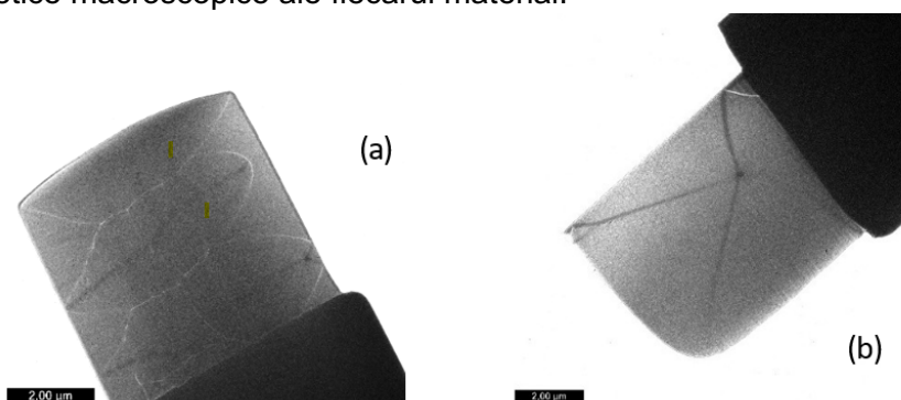
Fig. 15. Imagini LTEM ale domeniilor magnetice în microfire de (a) FeSiBCuNb și, respectiv, (b) CoFeSiB (diam. \sim 30 \mu\text{m} ) pentru un câmp magnetic aplicat H = 600 \text{ Oe} și un unghi de înclinare a eșantionului \alpha = 5^\circ .
