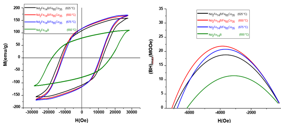
Fig. 11. Curbele de histeresis magnetic și curbele (BH)_{\max} vs. H pentru compacte Nd 2 Fe 14 B/Fe 65 Co 35 obținute prin SPS la diferite temperaturi (600, 625 și 650 °C, presiune 80 MPa, timp 10 min.), comparativ cu un compact Nd 2 Fe 14 B.
