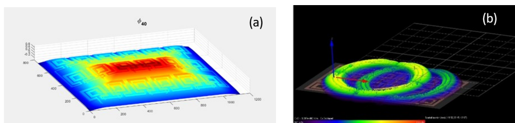
Fig. 18. (a) Diagrama de radiație rezultată SMMS, având 18 elemente, la frecvența de 178 MHz. (b) Distribuția curenților pentru excitația de tip undă plană la f = 178\text{MHz} (b)
