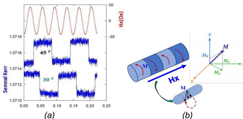
Fig. 1. (a) Dependența semnalului Kerr de unghiul de incidență și câmpul aplicat pentru un fir amorf de \text{Co}_{68,15}\text{Fe}_{4,35}\text{Si}_{12,5}\text{B}_{15} ( \Phi = 121 \mu\text{m} ) cu magnetostricțiune aproape zero. (b) Reprezentarea schematică a structurii de domenii magnetice în firul analizat.
