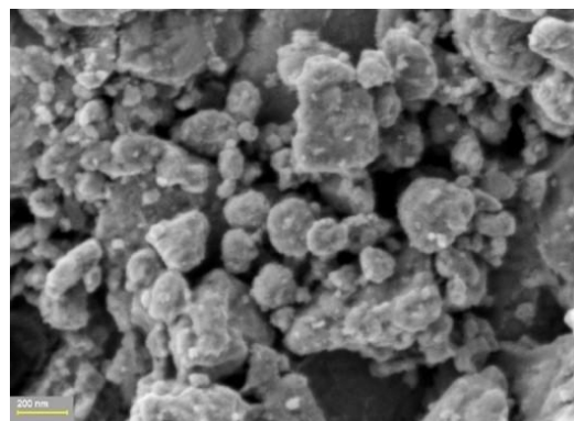
Fig. 10. Imagine SEM a pulberilor de Nd 14 Fe 80 B 6 obținute prin măcinare mecanică în atmosferă de aer.
